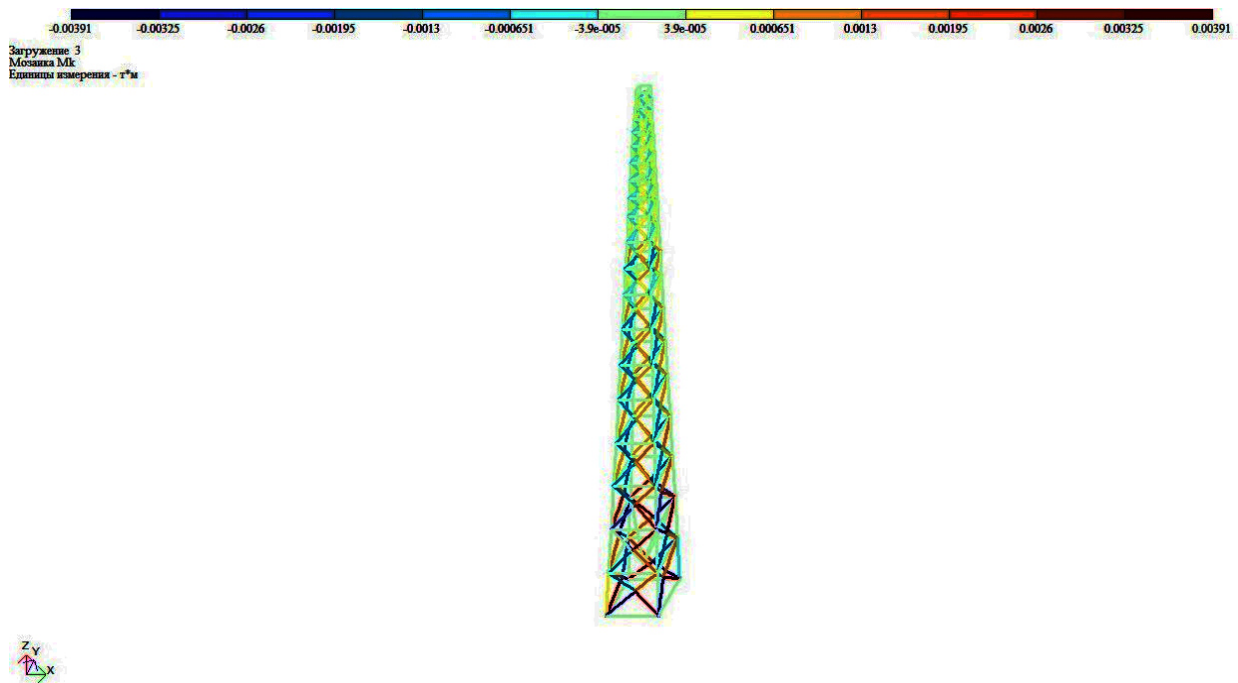
Рис. 4. Мозаїка розподілу згинальних моментів у вежі під вітровим навантаженням: a – без обледеніння та б – з обледенінням
