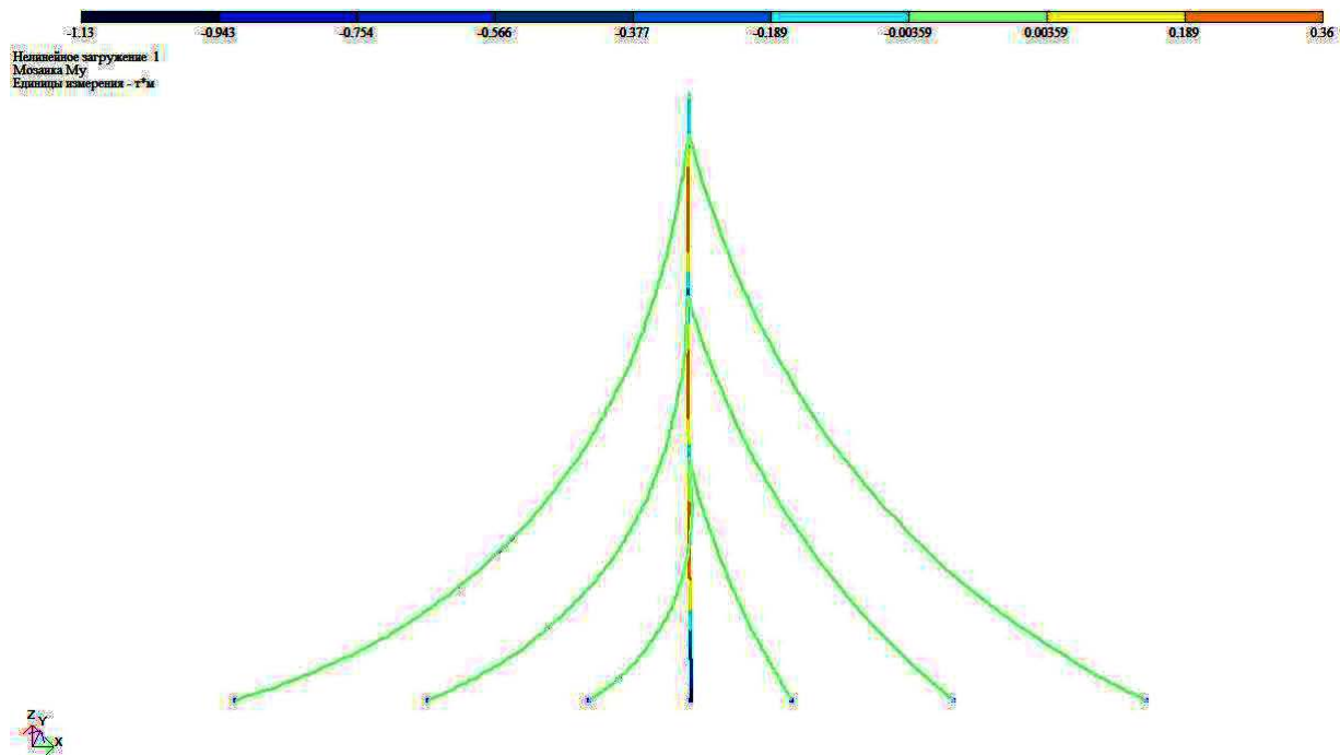
Рис. 3. Мозаїка розподілу згинальних моментів у щоглі під вітровим навантаженням: a – без обледеніння та б – з обледенінням
