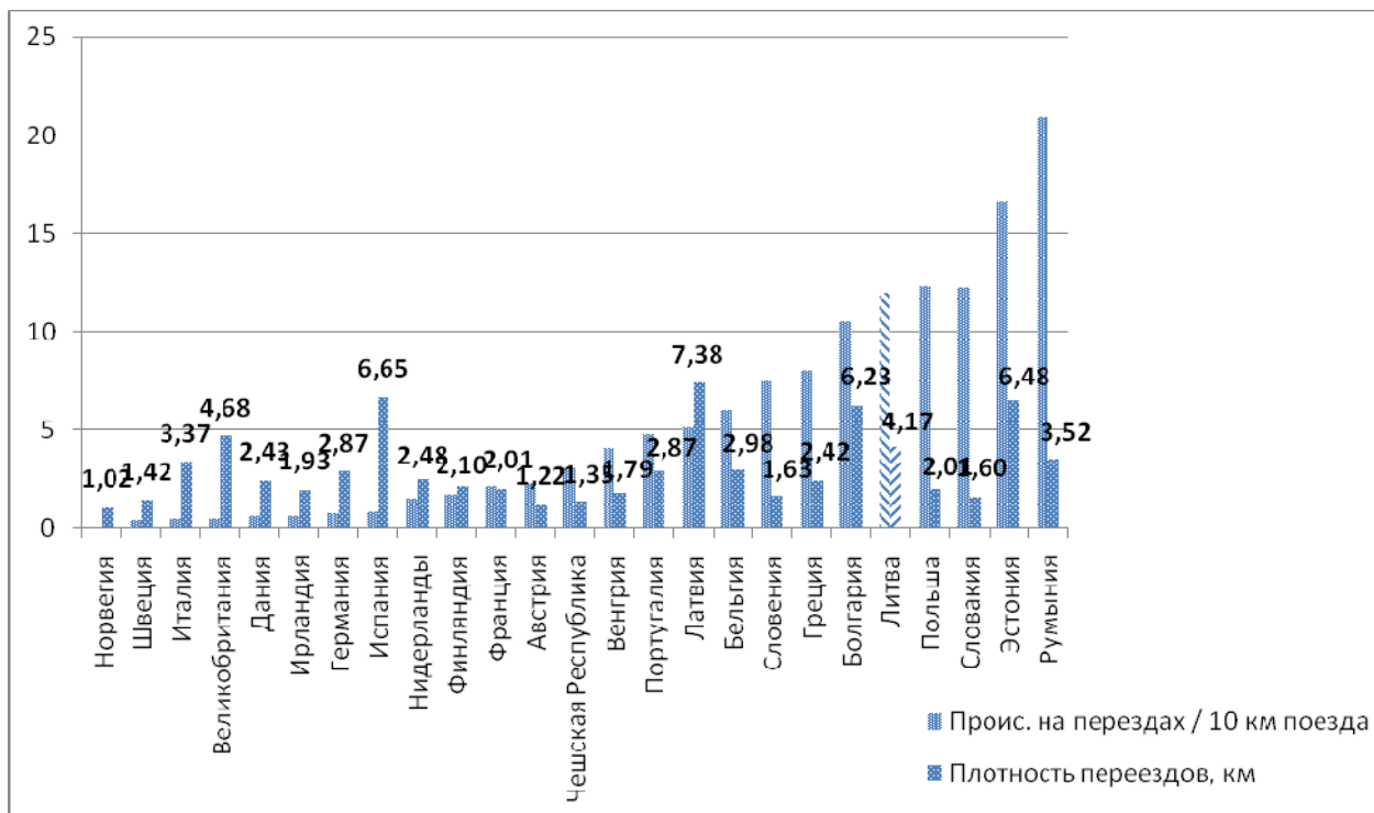
Рис. 1. Аварийность железнодорожного транспорта и плотность железнодорожных переездов в странах Европейского Союза и в Норвегии 2008 году
